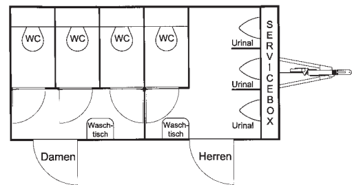
Raumeinteilung WC-Anhänger 5 m
